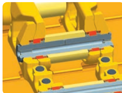
Boccole rotanti
