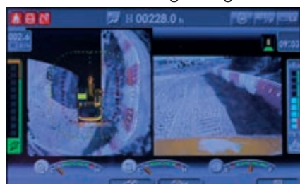
KomVision zeigt zusätzlich zu den verschiedenen Kameraansichten eine permanent verfügbare Draufsicht („Birdview“) an.
