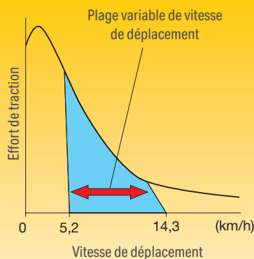
Commande de changement de vitesses variable avec plage de vitesse d'approche lente (gauche) et commutateur de limiteur de couple (TCS) variable (droite)
