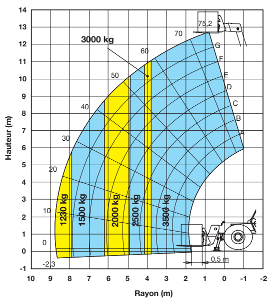
Sur stabilisateurs
