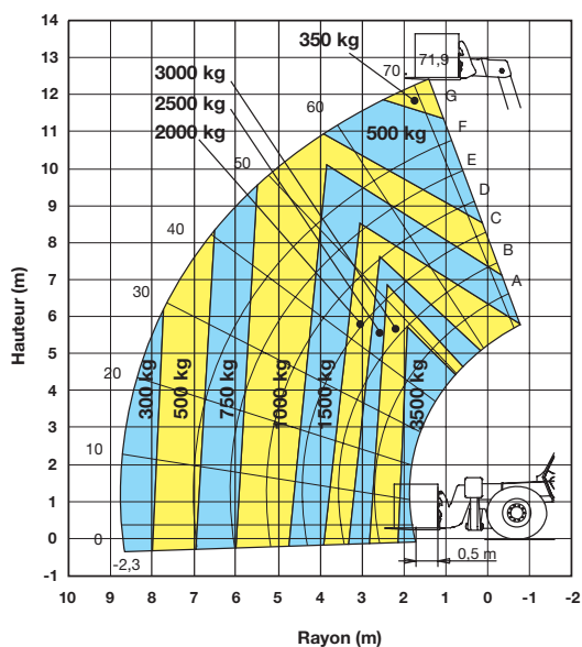
Sur pneus
