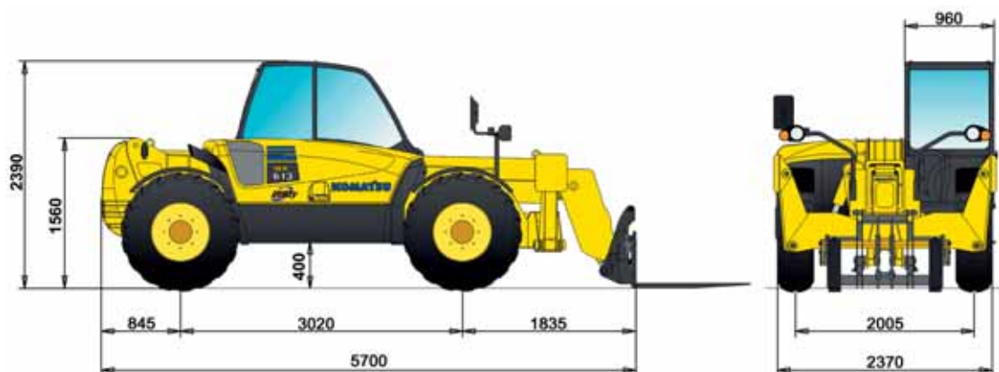
Sur pneus
